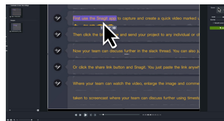
Erweiterte Cursoroptionen
